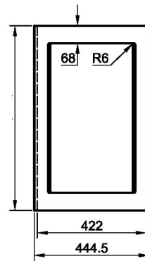
Стекло в выпуклую рамку
