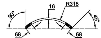
ВОГНУТАЯ РАМКА БЕЗ ЧЕТВЕРТИ
