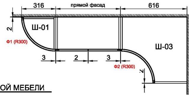
ВОГНУТАЯ РАМКА БЕЗ ЧЕТВЕРТИ
